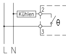
TRS 60 Schließer (NO)
