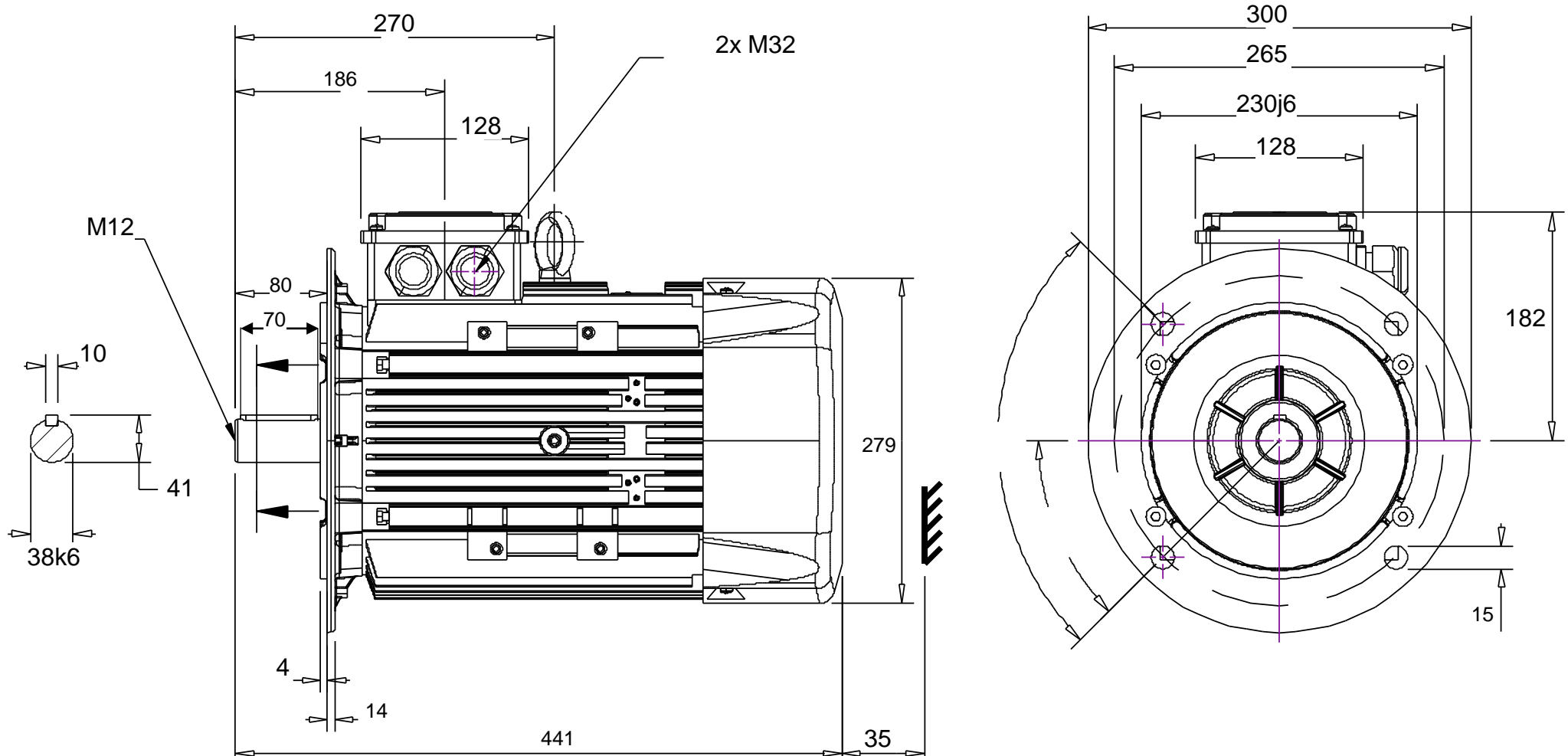
Maßblatt - #301956 - KTE 132 S 2 KT IE3 ULcsa in Angebot An151785 Position 1
