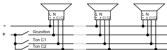
Anschlussbeispiel
